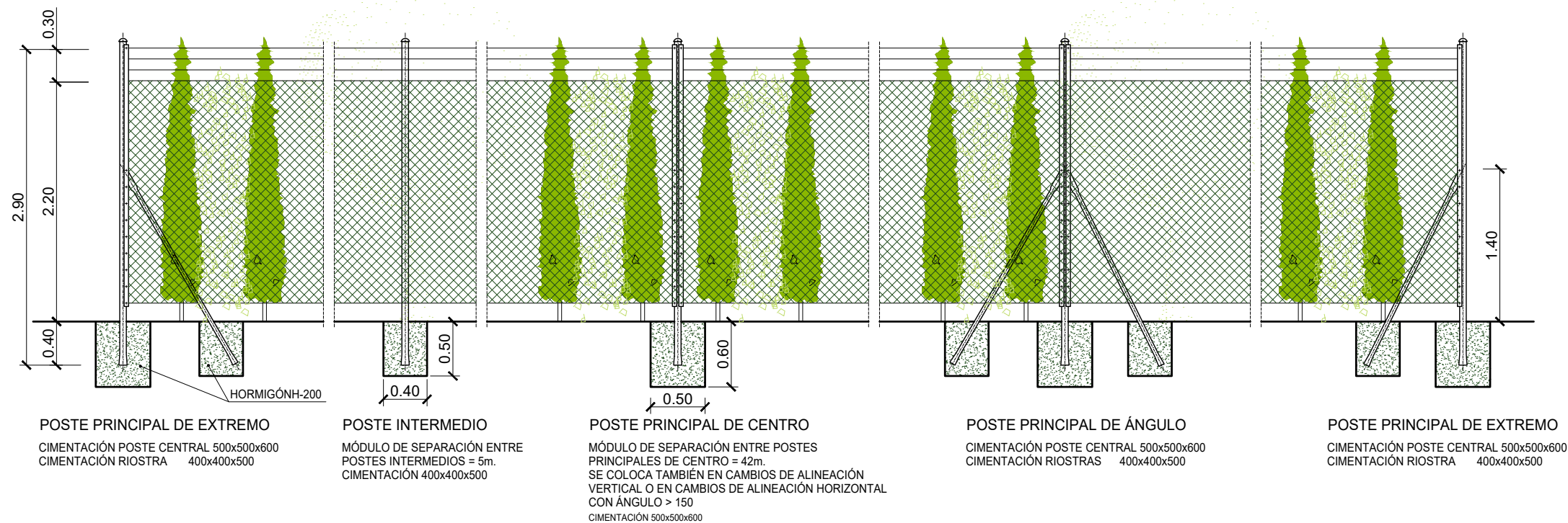
SECCIÓN TIPO
